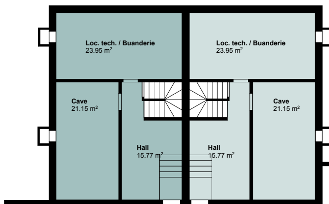
SOUS-SOL
