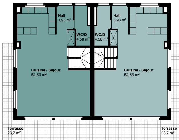
REZ-DE-CHAUSSEE
